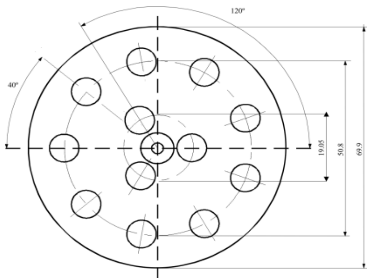
Рис. 2.4. Пенетрометр
