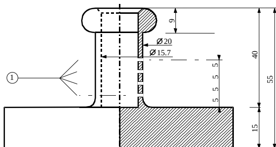
3. att. Dobs, vienā galā noslēgts, bronzas cilindrs; plānā un šķērsgrīzumā izmēri norādīti milimetros
