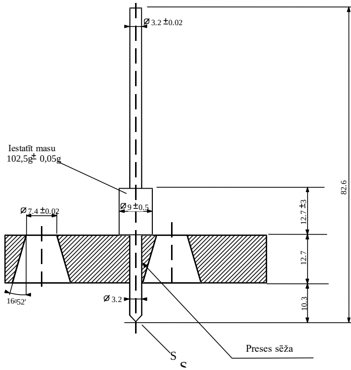
1. att. Penetrometrs
