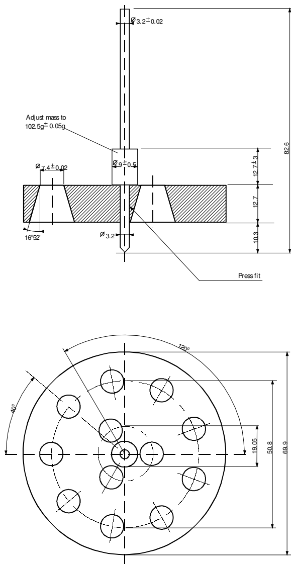
Рис. 2.4. Пенетромтр
