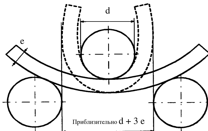
Схема испытания на изгиб
